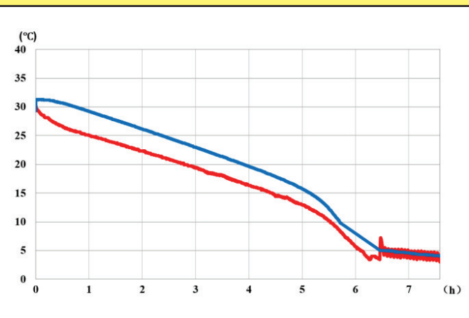
容器内的水温变化，当环境温度是 -35^{\circ}C 时，带有一个 0.1W/cm^2 ( 300W ) 的表面负载。 可以得出尽管加热功率增加，但罐的内部温度会继续缓慢下降。
