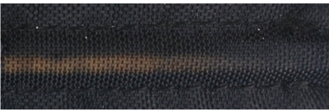
发热电缆在 220^{\circ}C 持续 1 小时：PA66 开始变色
